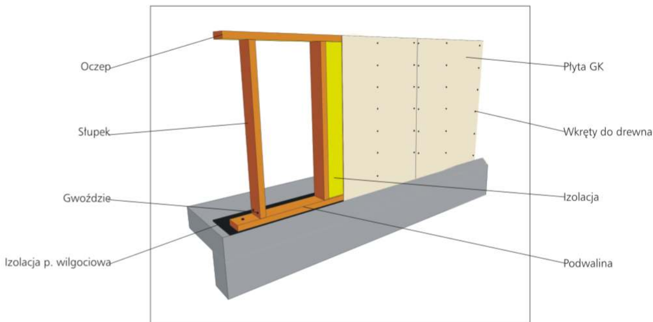
Rys.2 Ścianka działowa wykonana w systemie technologii konstrukcji drewnianej
