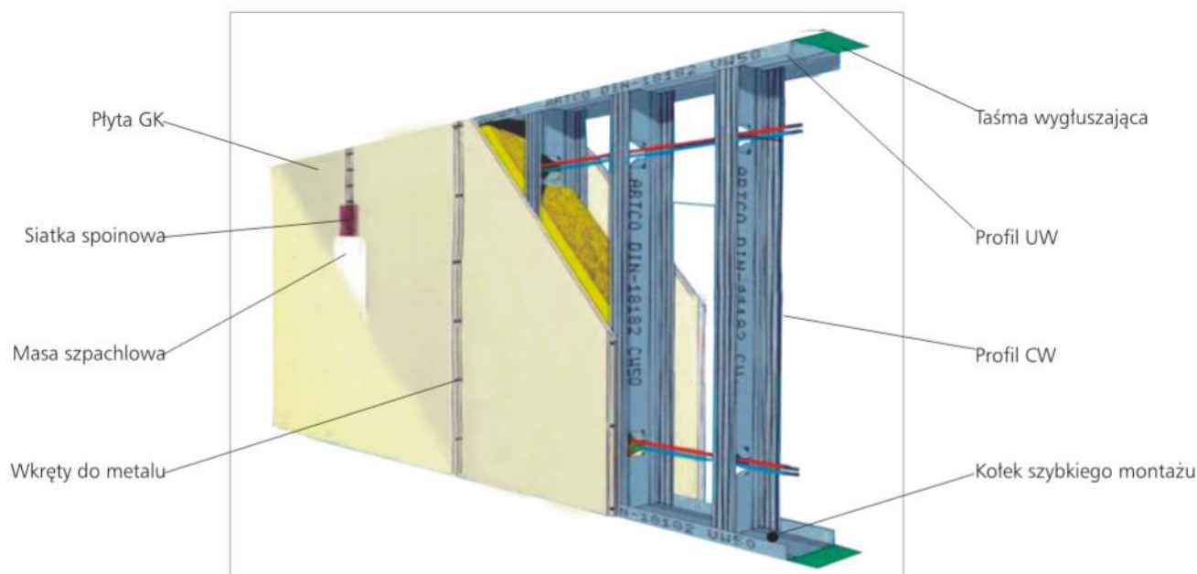
Rys.1 Ściana działowa z płyt GK na metalowej konstrukcji nośnej
